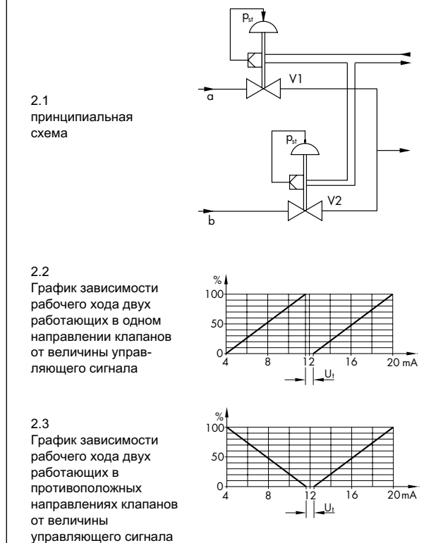
Рис. 2 · Два параллельных клапана, управляемых сигналом “y” в режиме работы с разбивкой диапазона регулирования
