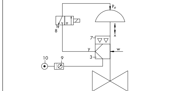
Рис. 3 · Пневматический клапан с дополнительным оснащением
