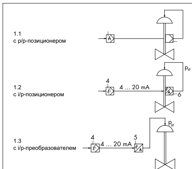
Рис. 1 · Схемы подключения пневматических приводов
