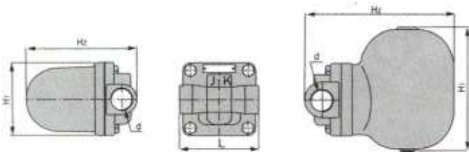
Сфероидный корпус Квадратная крышка Куполообразный корпус
